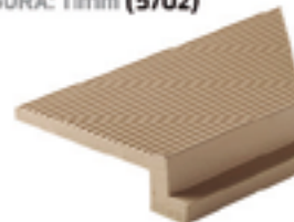
APOIO PARA GRELHA CANELADO 45° INTERNO ESQUERDO DIMENSÃO: 240/109 x 116 x 35 ESPESSURA: 11mm (5702)
