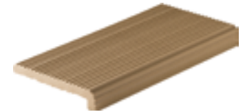
BORDA INFINITA CANELADA DIMENSÃO: 240mm/116mm x 25mm ESPESSURA: 9mm (5720)
